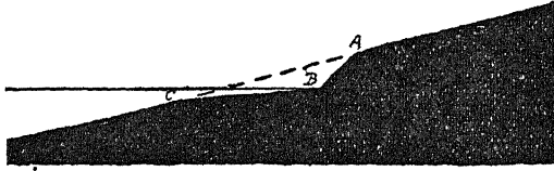
चित्र ६६—समुद्र से कट कर बना हुआ छज्जा
